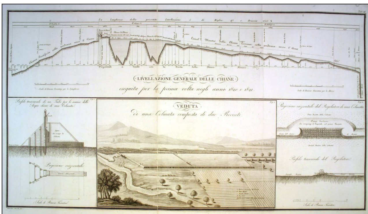
Livellazione generale delle Chiavari e veduta di una colmata composta di due recinti, in ALESSANDRO MANETTI, Carte idrauliche, cit., 1823.
